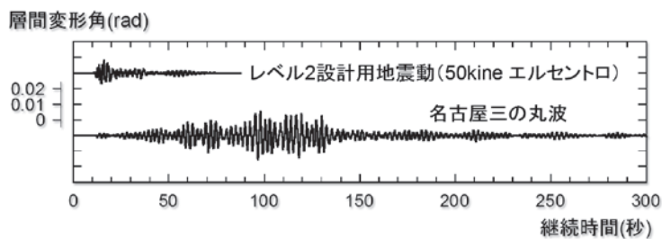
図1 実験による骨組の層間変形角履歴
