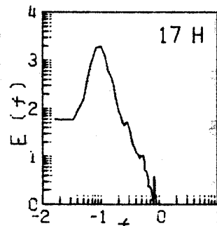
図4. 波浪のパワースペクトルの例示
