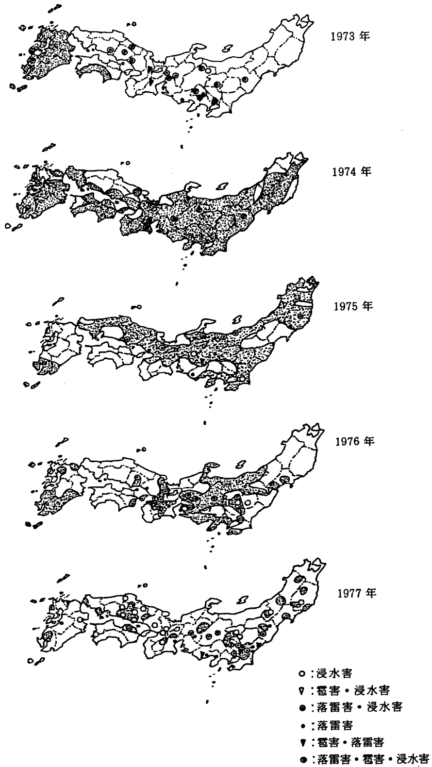
図3 (2) 年別の雷雨の被害分布(7月)。
