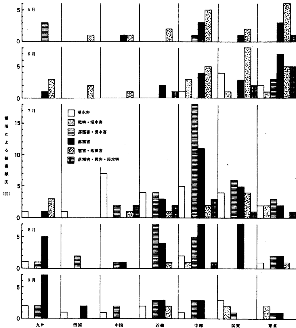
図2 地方別の雷雨による被害の頻度 (1973年～1977年)。
