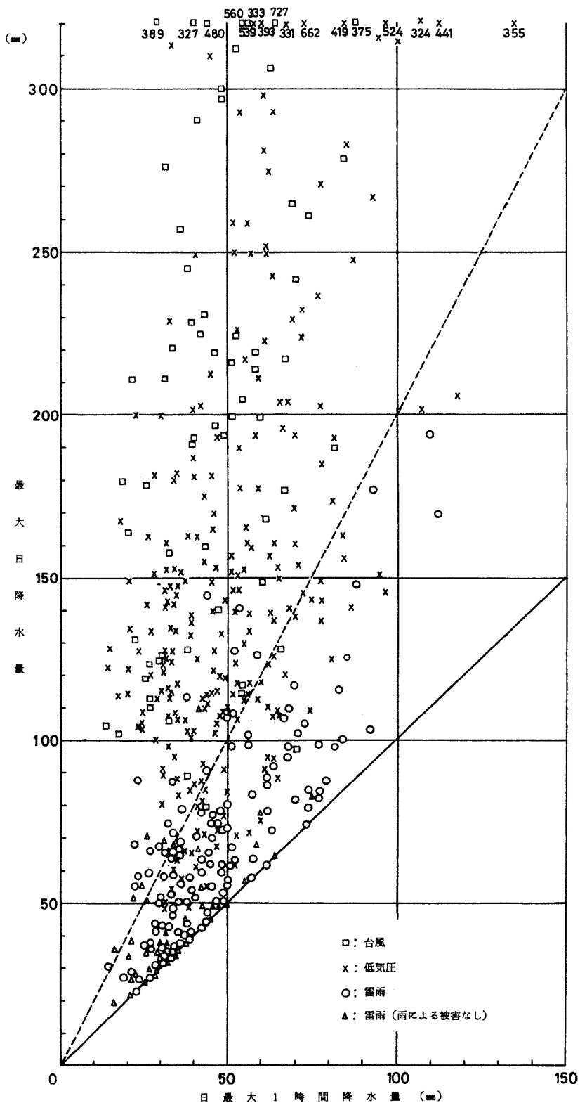
図7 最大日降水量と日最大1時間降水量の関係。日降水量が320mmを越える場合には、記号を320mm上に記入し、降水量を数字で示した。実線は日最大1時間降水量と最大日降水量が等しい場合を示す。破線は最大日降水量が日最大1時間降水量の2倍であることを示す。
