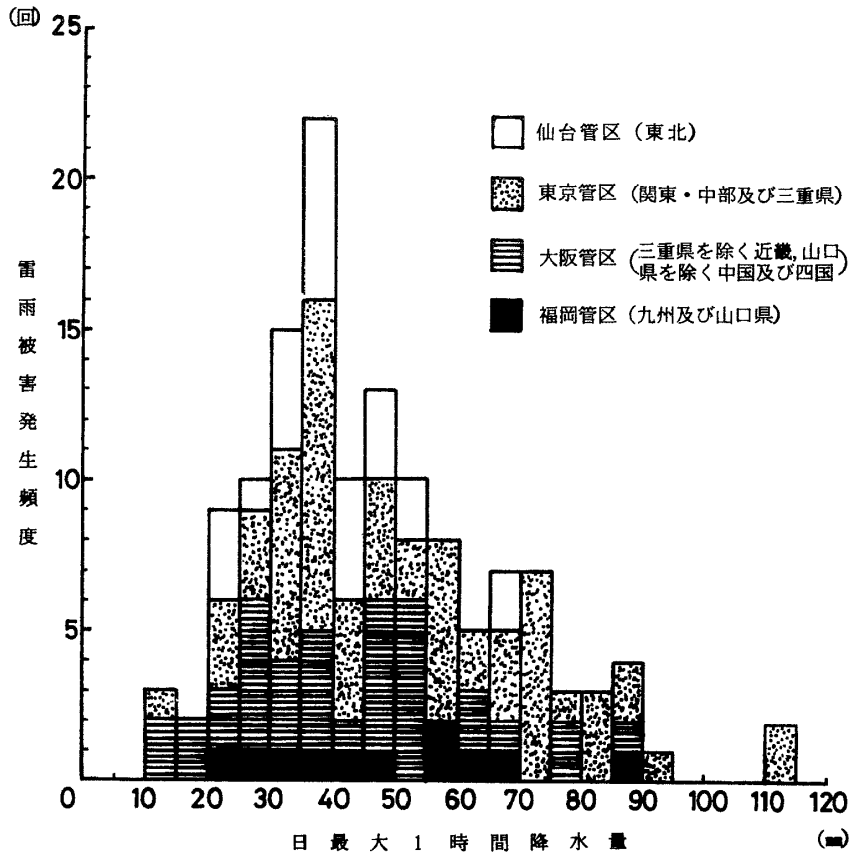
図9 1時間降水量に対する雷雨被害発生頻度 (1973年～1977年)。
