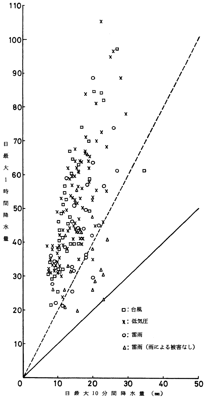
図 8 日最大1時間降水量と日最大10分間降水量の関係。実線は日最大1時間降水量と日最大10分間降水量が等しい場合を示す。破線は日最大1時間降水量が日最大10分間降水量の2倍であることを示す。
