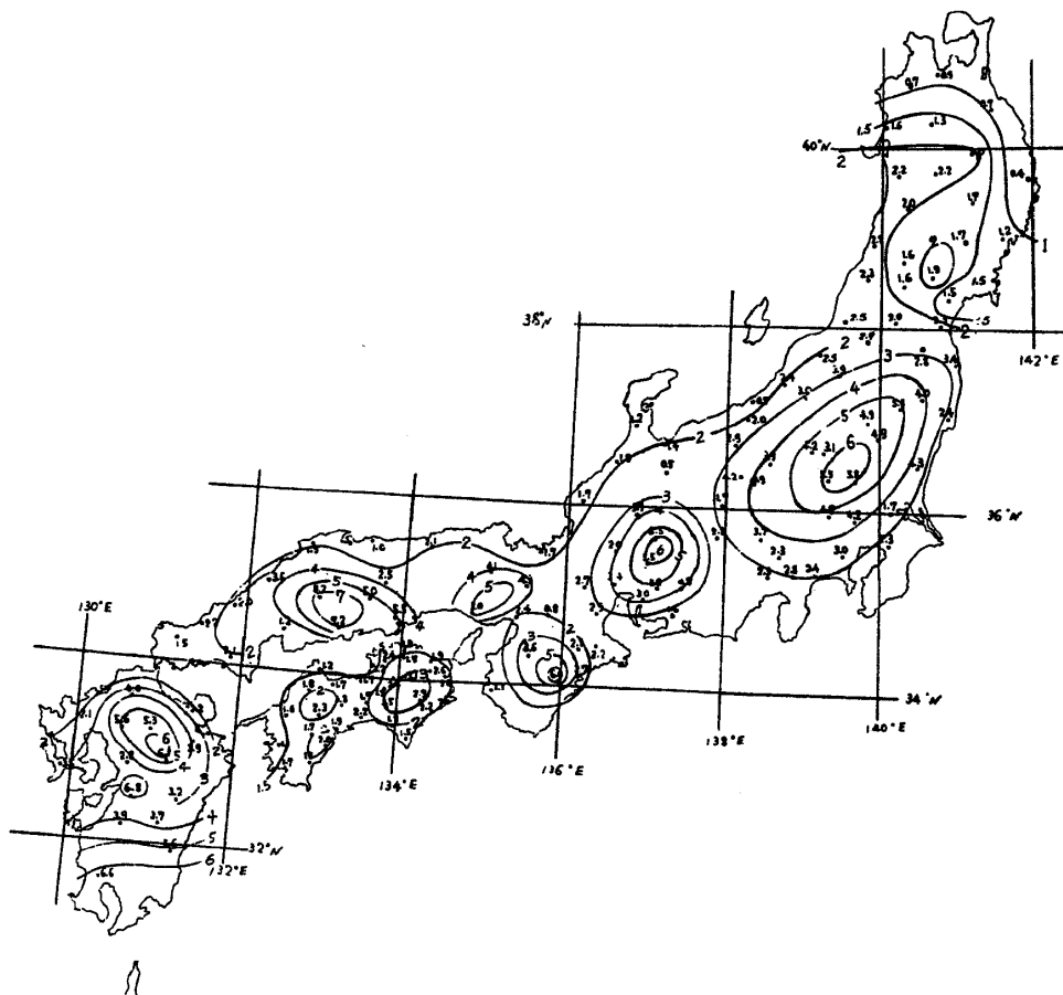
図6 雷放電ひん度分布図(雷害事故調査委員会(1976)による)。昭和39年～昭和49年、11年平均、6月～9月。
