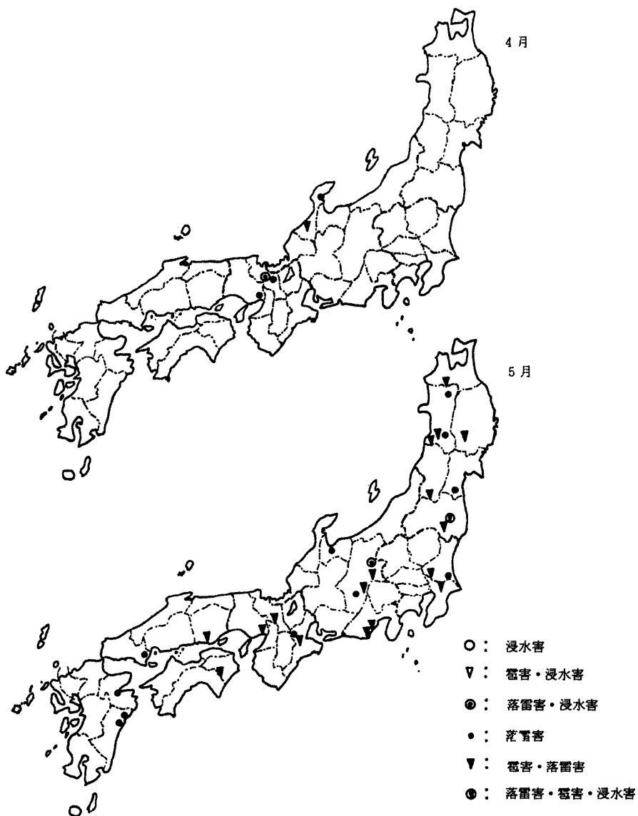
図1 雷雨の被害分布 (1973年～1977年)
