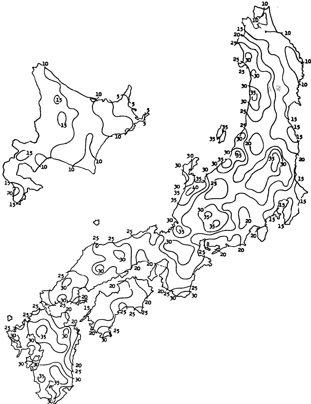
図5 年間雷雨日数分布図(雷雨10年報(昭和29年～昭和38年)による)。
