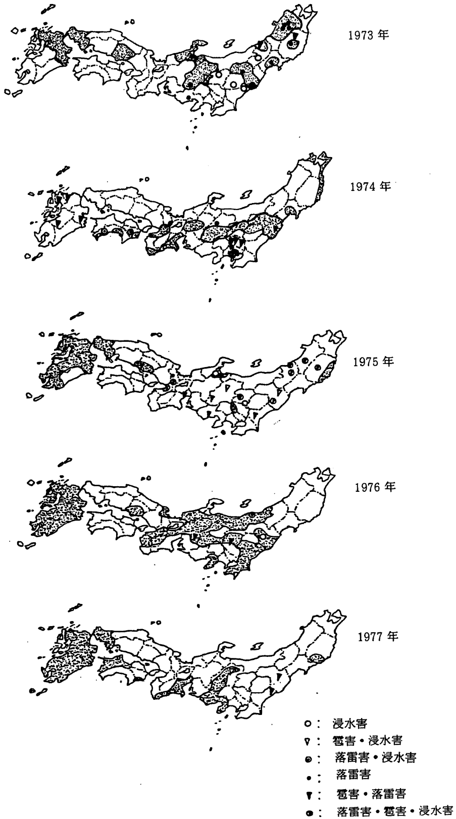
図3 (1) 年別の雷雨の被害分布(6月)。小さな点々で示した部分は雨による被害を受けた地区 (気象要覧から転載)
