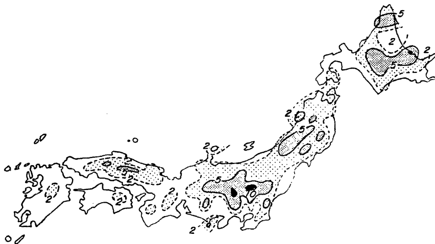
図4 暖候期の雷雨日数分布図 (Omoto (1967) による)。1954年～1964年、6月～9月について。
