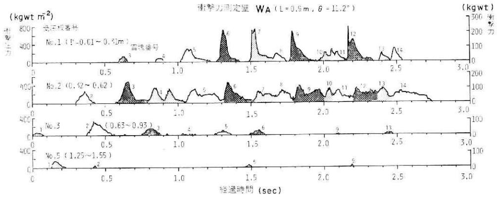
図10 測定壁 WA で測定した衝撃圧力 (横軸は, 衝撃力を感知し始めた時点を中心とした) Fig.10 Impact forces measured at the wall WA.
