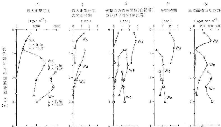
図13 各測定壁に及ぼされた衝撃圧力の作用状況 Fig. 13 Vertical distribution of the impact forces.
