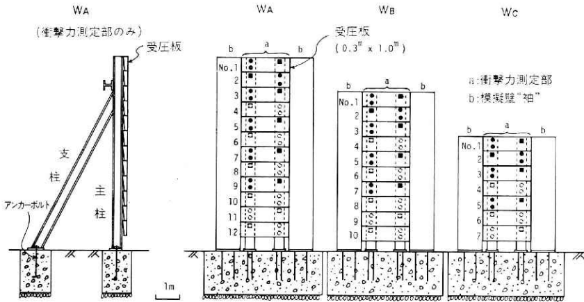
図3 衝撃力測定壁 ○, □: ロードセル取付け可能箇所 (○水平成分測定用, □鉛直成分測定用) 黒塗りはロードセルを実際に取付けた箇所
