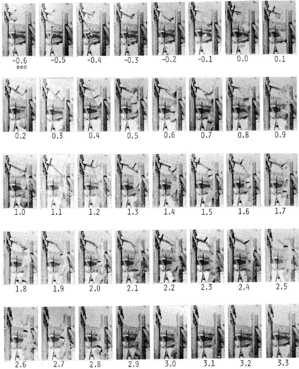
写真 7 屋根 R_A から滑落する雪塊が測定壁 W_A に衝突する状況. 下の数字は写真番号を示すと同時に経過時間 (単位: 秒) を表わし, 図10の時間軸に合致させてある. Photo. 7 Sequence of the movements of the snow blocks sliding down from the roof R_A . Numbers show the time from beginning of the collision in second and correspond to the time graduations on the abscissa in Figs. 10~12.
