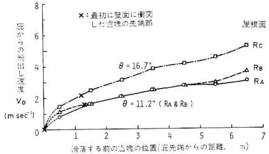
図7 庇(ひさし)を離れる時の雪塊の飛出し速度
