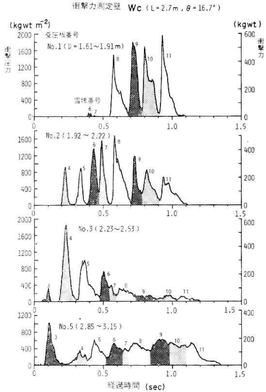
図12 測定壁 Wc で測定した衝撃圧力 (横軸は、衝撃力を感じし始めた時点と原点とした) Fig. 12 Impact forces measured at the wall Wc.
