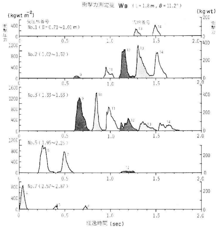
図11 測定壁 WB で測定した衝撃圧力 (横軸は, 衝撃力を感知し始めた時点を中心とした) Fig.11 Impact forces measured at the wall WB.
