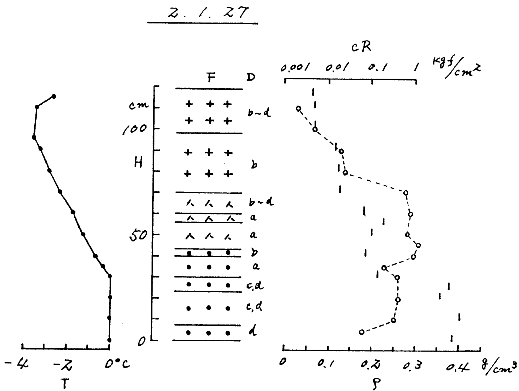
図3 積雪断面観測図 (長岡, 平成元年12月~平成2年2月) (つづき) Fig. 3 Vertical profile of physical properties of snow cover in Nagaoka (Dec.1989 - Feb.1990) . (continued)
