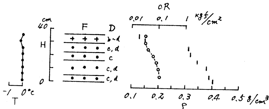
図3 積雪断面観測図 (長岡, 平成元年12月~平成2年2月) (つづき) Fig. 3 Vertical profile of physical properties of snow cover in Nagaoka (Dec.1989 - Feb.1990) . (continued)
