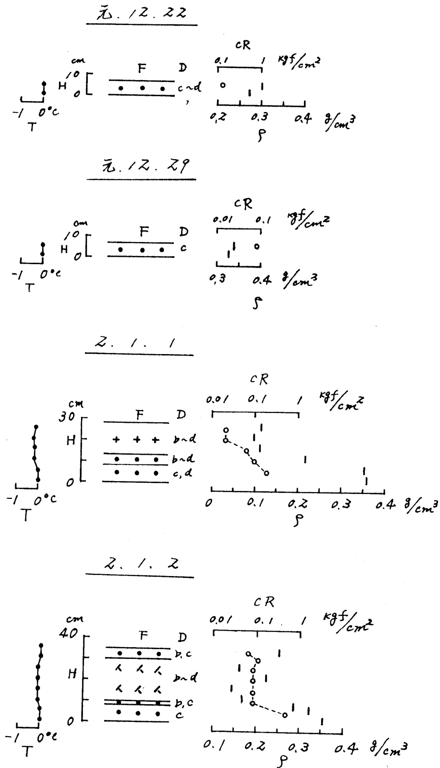
図3 積雪断面観測図 (長岡, 平成元年12月~平成2年2月) (つづき) Fig. 3 Vertical profile of physical properties of snow cover in Nagaoka (Dec.1989 - Feb.1990) . (continued)
