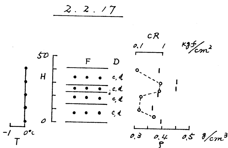
図3 積雪断面観測図 (長岡, 平成元年12月~平成2年2月) (つづき)
