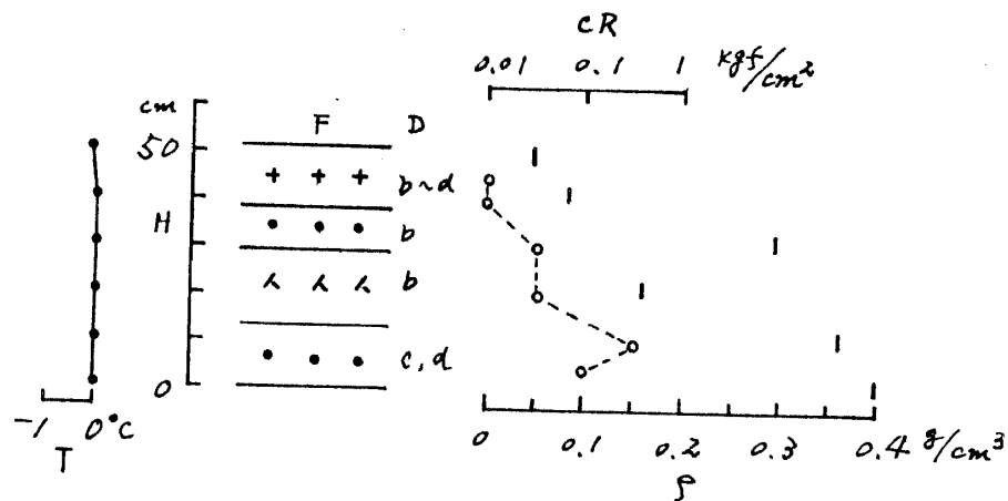
図3 積雪断面観測図 (長岡, 平成元年12月~平成2年2月) (つづき) Fig. 3 Vertical profile of physical properties of snow cover in Nagaoka (Dec.1989 - Feb.1990) . (continued)
