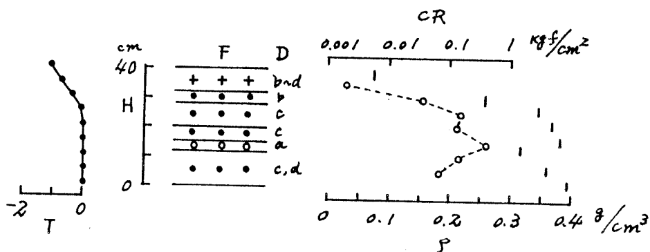
図3 積雪断面観測図 (長岡, 平成元年12月~平成2年2月) (つづき) Fig. 3 Vertical profile of physical properties of snow cover in Nagaoka (Dec.1989-Fib.1990) . (continued)
