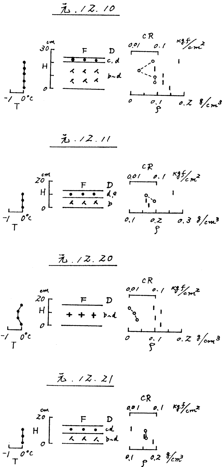
図3 積雪断面観測図 (長岡, 平成元年12月~平成2年2月) (つづき) Fig. 3 Vertical profile of physical properties of snow cover in Nagaoka (Dec.1989 - Feb.1990) . (continued)
