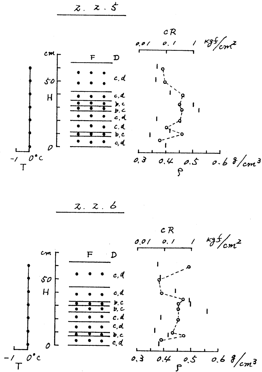
図3 積雪断面観測図 (長岡, 平成元年12月~平成2年2月) (つづき) Fig. 3 Vertical profile of physical properties of snow cover in Nagaoka (Dec.1989 - Feb.1990) . (continued)
