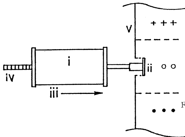
図6 カナディアンハードネスゲージの測定方法
