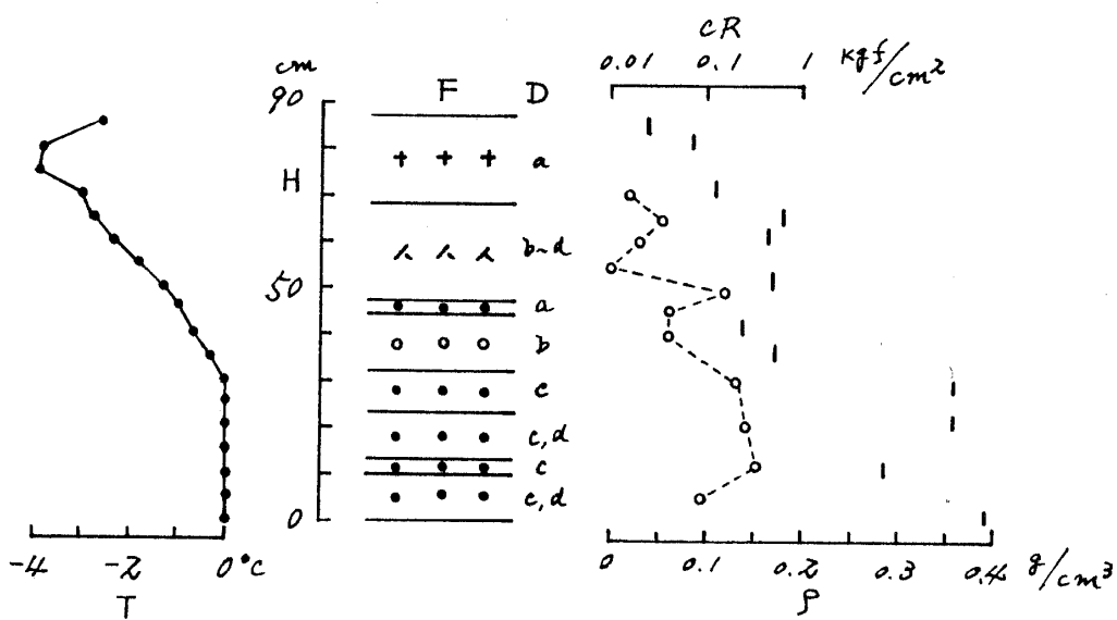
図3 積雪断面観測図 (長岡, 平成元年12月~平成2年2月) (つづき) Fig. 3 Vertical profile of physical properties of snow cover in Nagaoka (Dec.1989-Feb.1990) . (continued)
