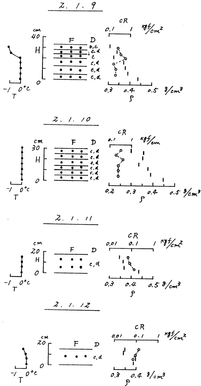
図3 積雪断面観測図 (長岡, 平成元年12月~平成2年2月) (つづき)
