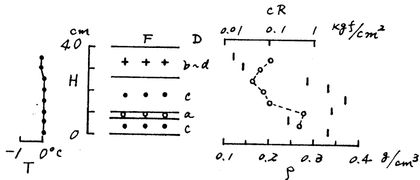
図3 積雪断面観測図 (長岡, 平成元年12月~平成2年2月) (つづき) Fig. 3 Vertical profile of physical properties of snow cover in Nagaoka (Dec.1989 - Feb.1990) . (continued)
