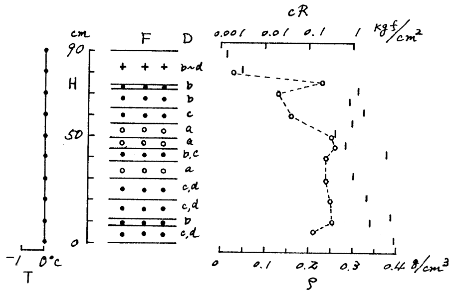
図3 積雪断面観測図 (長岡, 平成元年12月~平成2年2月) (つづき) Fig. 3 Vertical profile of physical properties of snow cover in Nagaoka (Dec.1989-Feb.1990) . (continued)
