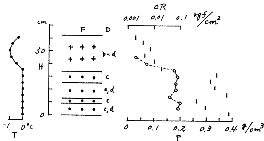
図3 積雪断面観測図 (長岡, 平成元年12月~平成2年2月) (つづき) Fig. 3 Vertical profile of physical properties of snow cover in Nagaoka (Dec.1989 - Feb.1990) . (continued)
