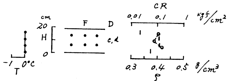
図3 積雪断面観測図 (長岡, 平成元年12月~平成2年2月) (つづき) Fig. 3 Vertical profile of physical properties of snow cover in Nagaoka (Dec.1989-Feb.1990) . (continued)
