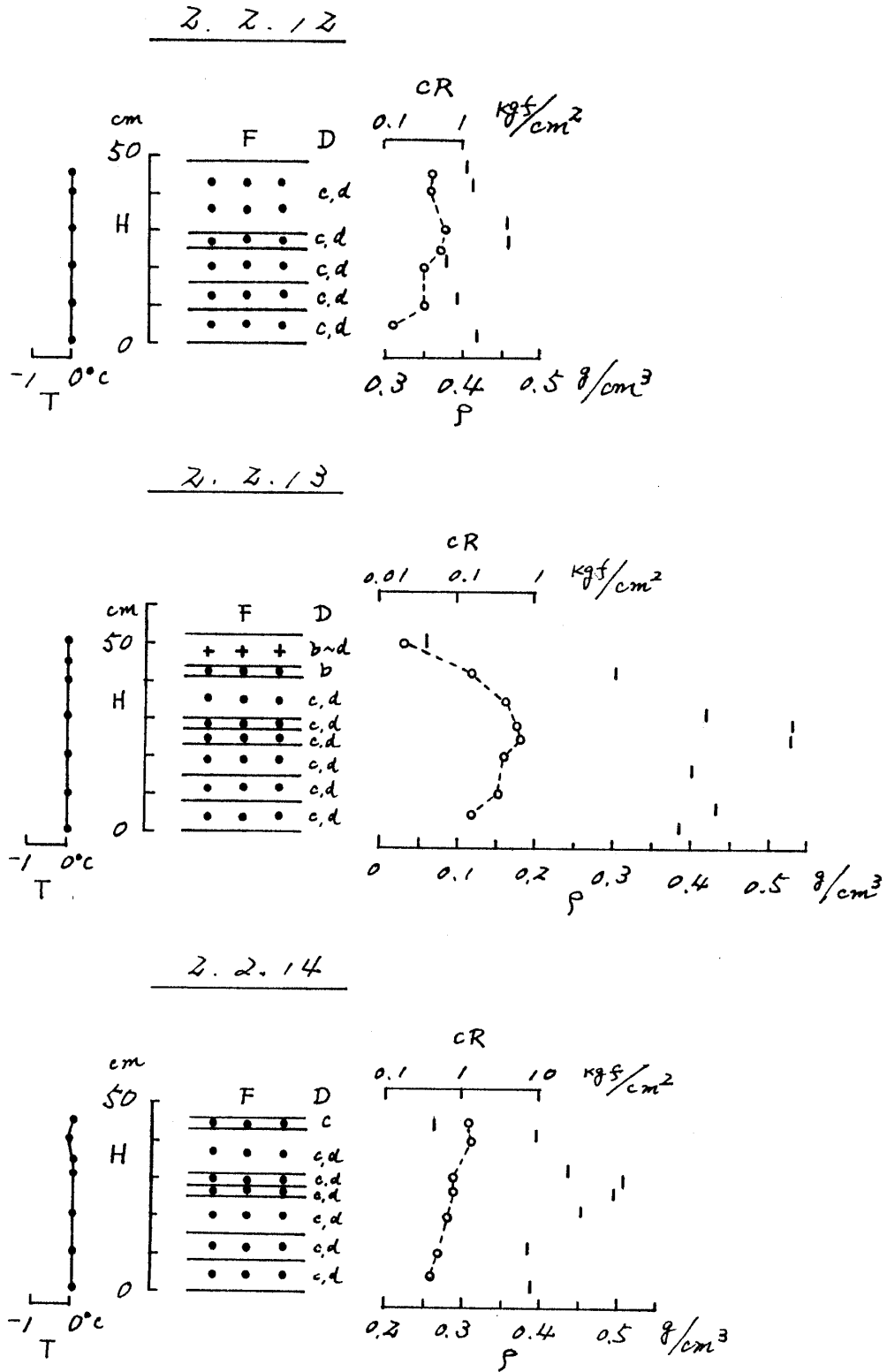
図3 積雪断面観測図 (長岡, 平成元年12月~平成2年2月) (つづき) Fig. 3 Vertical profile of physical properties of snow cover in Nagaoka (Dec.1989 - Feb.1990) . (continued)
