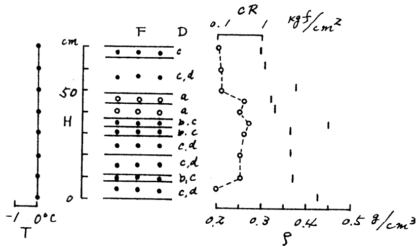
図3 積雪断面観測図 (長岡, 平成元年12月~平成2年2月) (つづき) Fig. 3 Vertical profile of physical properties of snow cover in Nagaoka (Dec.1989~Fib.1990) . (continued)
