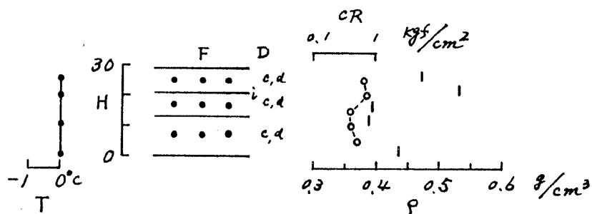
図3 積雪断面観測図 (長岡, 平成元年12月~平成2年2月) (つづき) Fig. 3 Vertical profile of physical properties of snow cover in Nagaoka (Dec.1989 - Feb.1990) . (continued)
