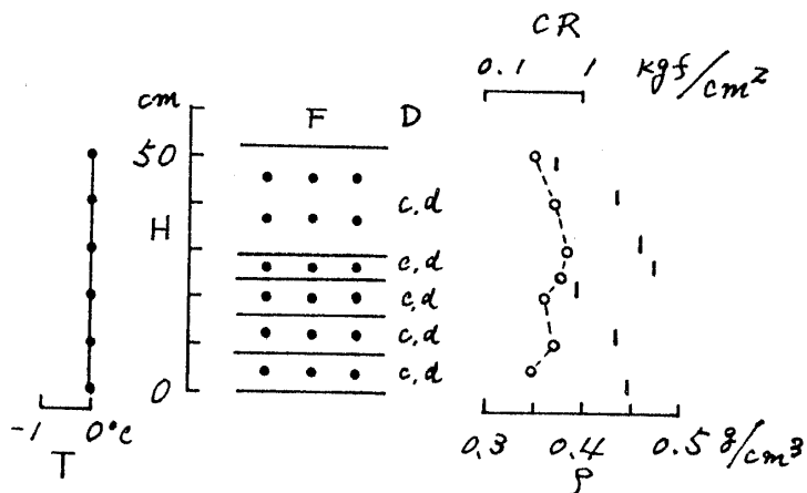
図3 積雪断面観測図 (長岡, 平成元年12月~平成2年2月) (つづき) Fig. 3 Vertical profile of physical properties of snow cover in Nagaoka (Dec.1989 - Feb.1990) . (continued)
