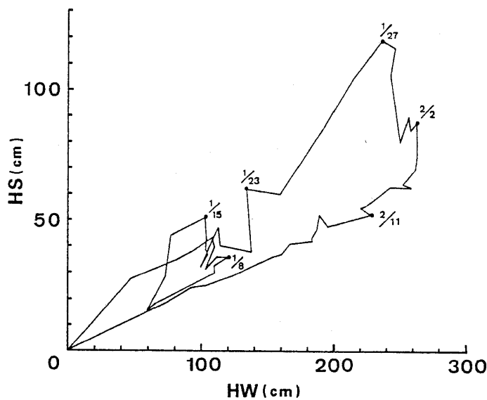
図4 積雪の深さと積雪相当水量の循環曲線図 (1990年1月1日~1990年2月23日)
