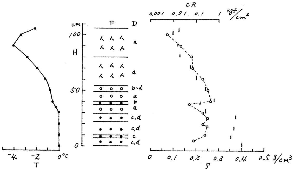
図3 積雪断面観測図 (長岡, 平成元年12月~平成2年2月) (つづき) Fig. 3 Vertical profile of physical properties of snow cover in Nagaoka (Dec.1989 - Feb.1990). (continued)
