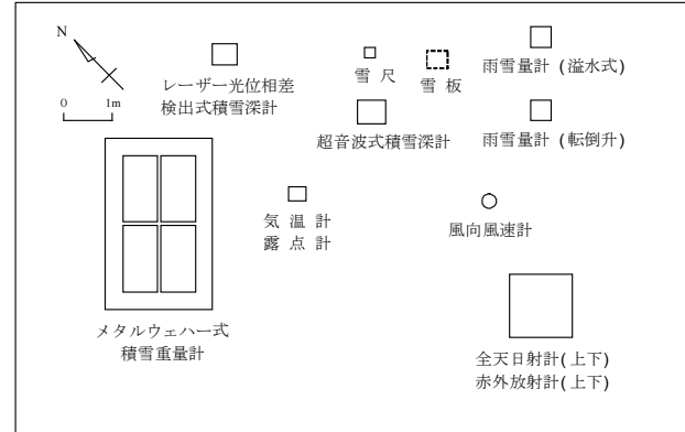
図4 第2気象観測露場(15m×20m)の計測器配置図 Fig. 4 Horizontal distribution of sensors in the No.2 meteorological field(15m×20m).
