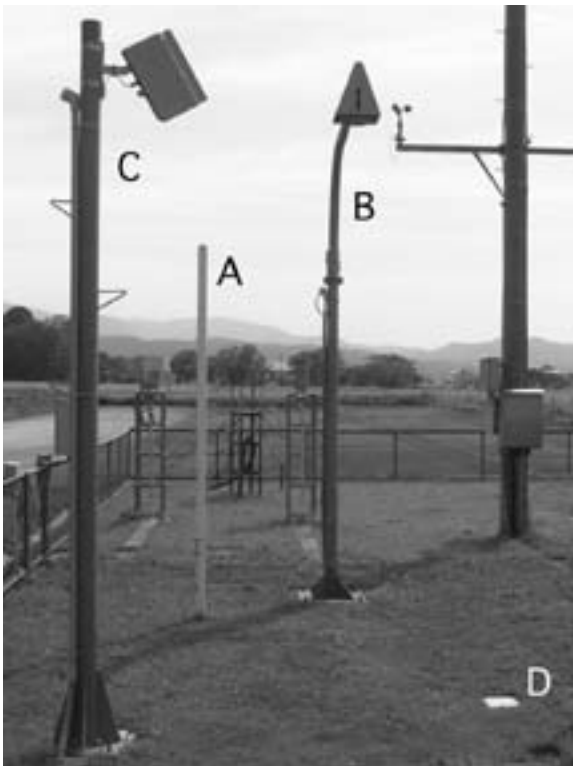
図5 雪尺(A)、超音波式積雪深計(B)及びレーザー光波位相差検出式積雪深計(C)とその0レベル基準面(D)。
