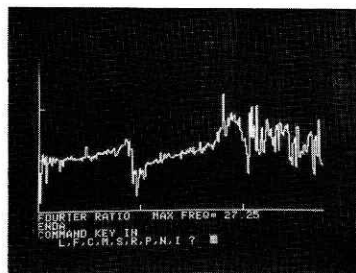
フーリエ比
