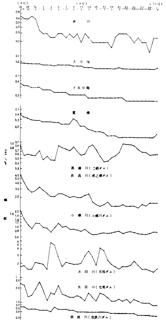
図-9 各地点の流量変化
