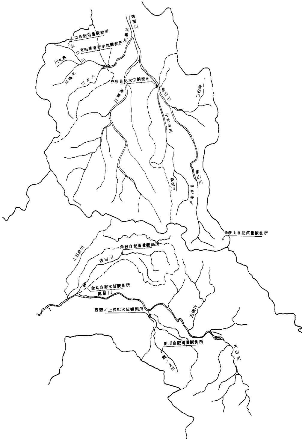
図 - 1 1 水位雨量観測所配置図
