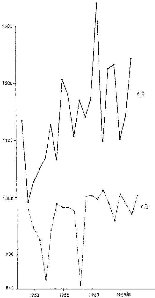
図-6 長崎の蒸発散能
