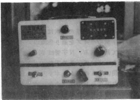
写真3 降雪強度計の増幅器 Amplifier of snowfall intensity-meter.
