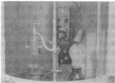
写真2 受雪部の内部 Inside view of the snow collecting instrument.
