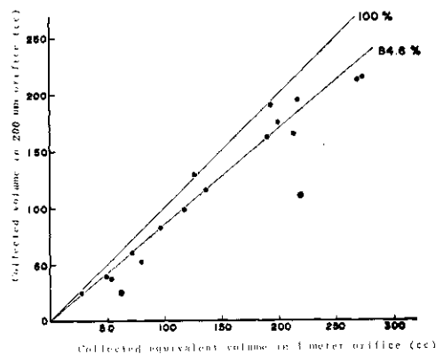
図7 口径1mと200mmの受雪器に入った雪の量の比較
