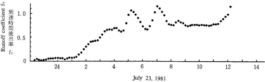
図4 E流域における豪雨時の到達時間流出率 f_r と貯留高 S の時間変化。
