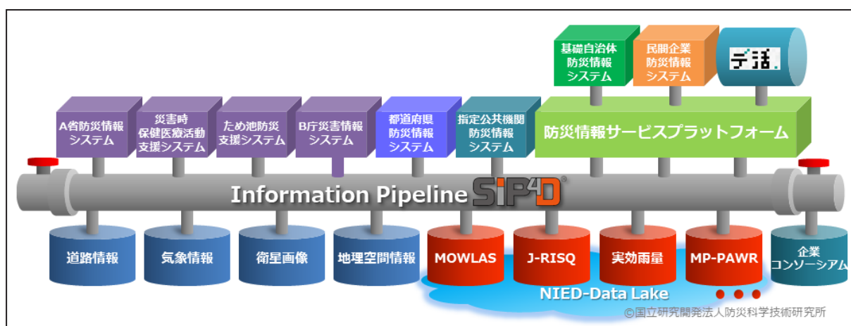
図 1 SIP4D の概要 (SIP4D のホームページ [2] より)
