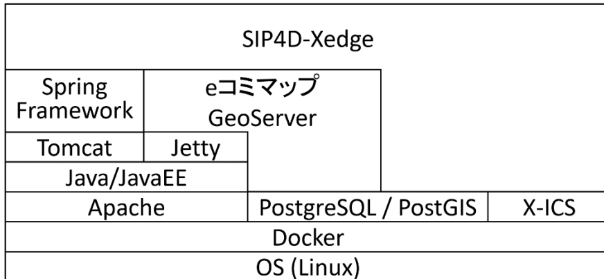
図 3 ソフトウェア構成図
