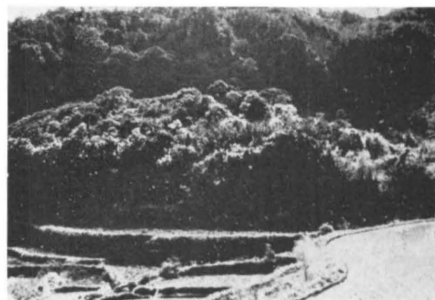
写真4 古い地すべりにより玄武岩の移動岩塊からなる小丘
