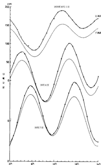
図1 平塚沖波浪観測塔で測定された相対潮位(実線)と予測値(破線)
