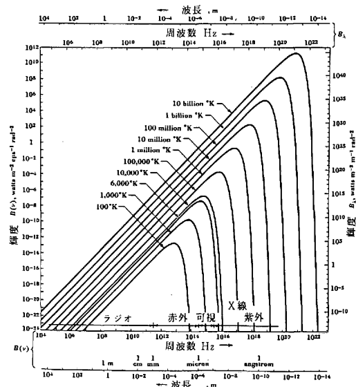
図1 プランクの法則から導かれる輻射スペクトルの分布を幾つかの温度の場合に示した。
