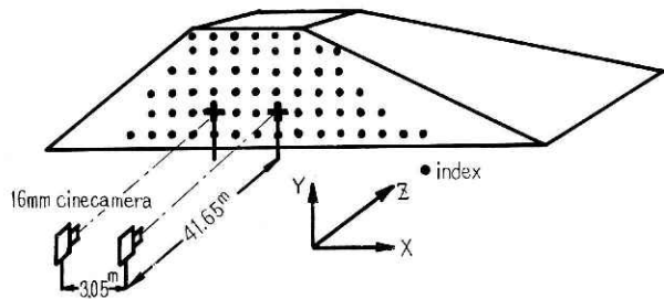
図 13 撮影機配置図 Fig. 13 Outline of the photographing
