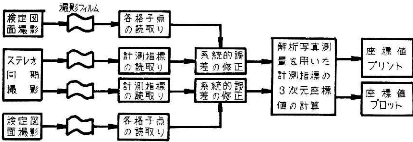
図 12 解析写真測量システム Fig. 12 System of the analytical photogrammetry
