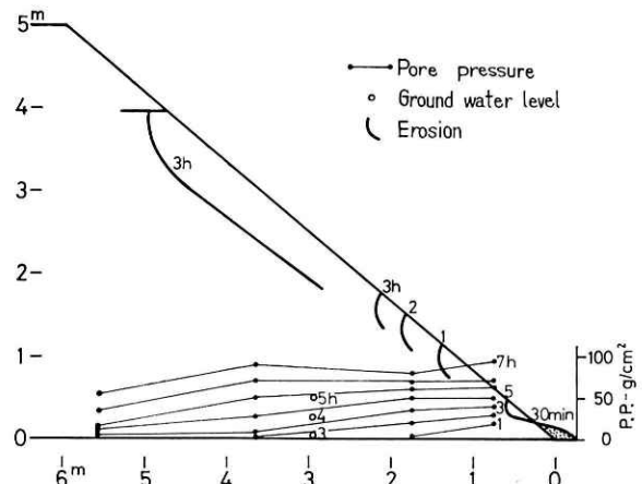
図 9 間ゲキ圧の変化と浸食の進行状況 (40° 斜面)
