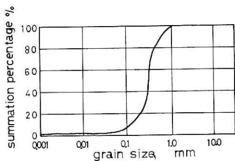
図 3 粒度分布曲線 Fig. 3 Grain size distribution curve
