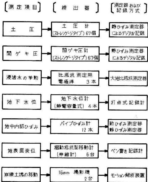
図 2 計測システム Fig. 2 Outline of measurement
